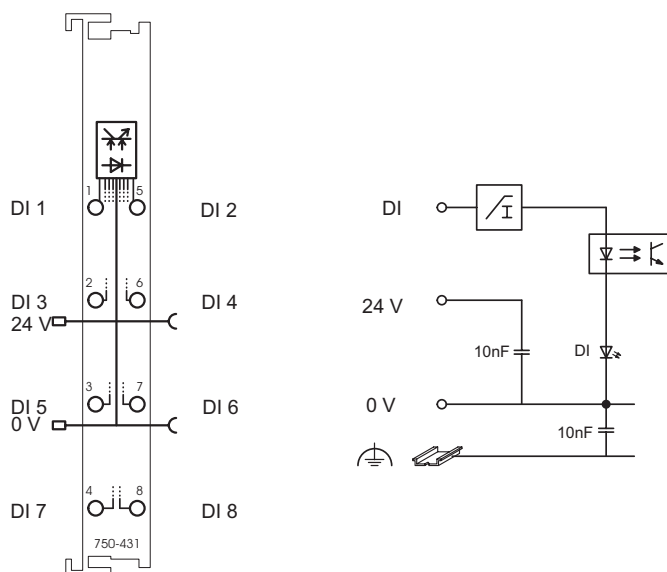
Abb. 2.1.1-3: 8-Kanal Digital Eingangsklemme 750-431
