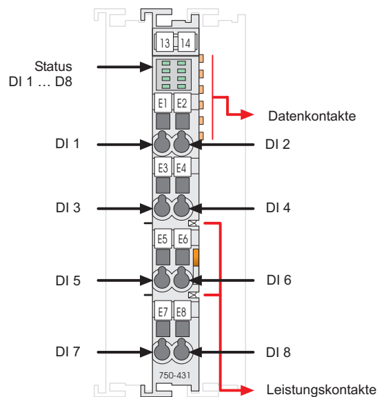
Abb. 2.1.1-1: 8-Kanal Digital Eingangsklemme 750-431
